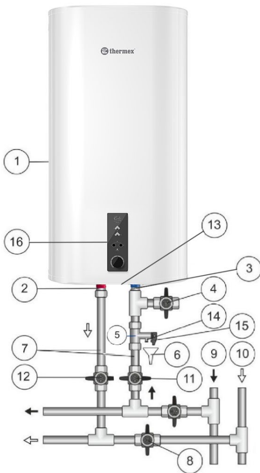
Рисунок 1. Схема подключения ЭВН к водопроводу
